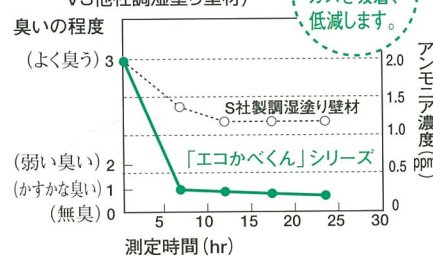
アンモニア濃度と臭気の経時変化比較 (「エコかべくん」シリーズ VS 他社調湿塗り壁材)
