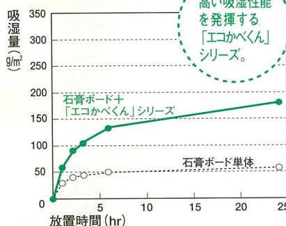
吸放湿性能(吸湿量)比較
