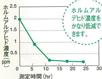
ホルムアルデヒド濃度の経時変化 (「エコかべくん」シリーズ)
