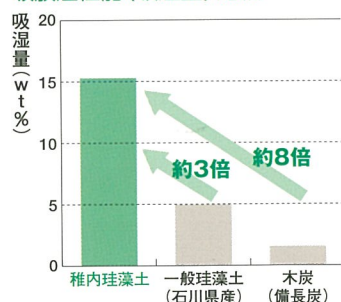
吸放湿性能(吸湿量)比較
